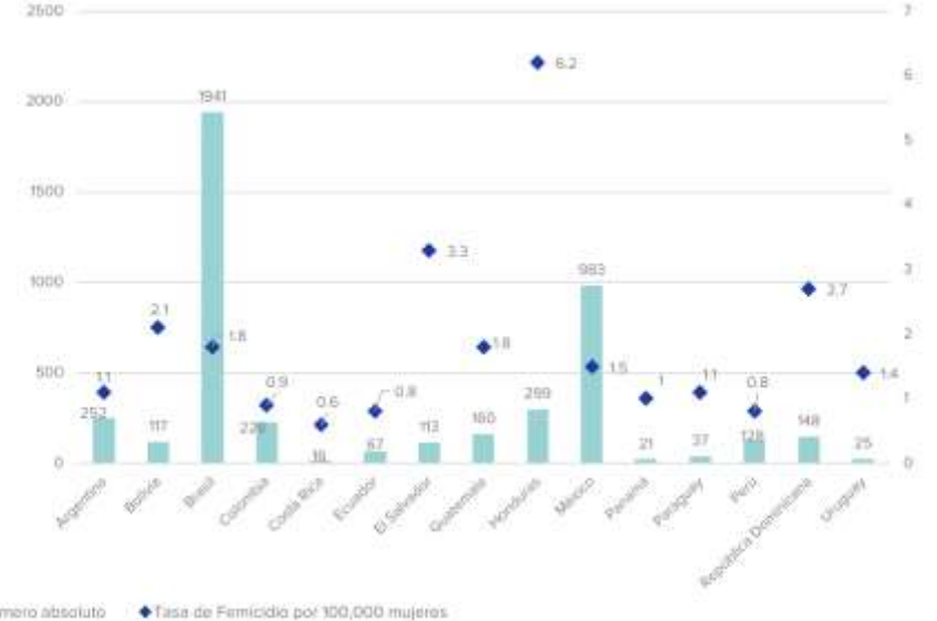
Femicidio o femicidios, en países seleccionados de Centroamérica, República Dominicana y el resto de América Latina último año 2019 (En números absolutos y tasas por cada 100.000 mujeres)
