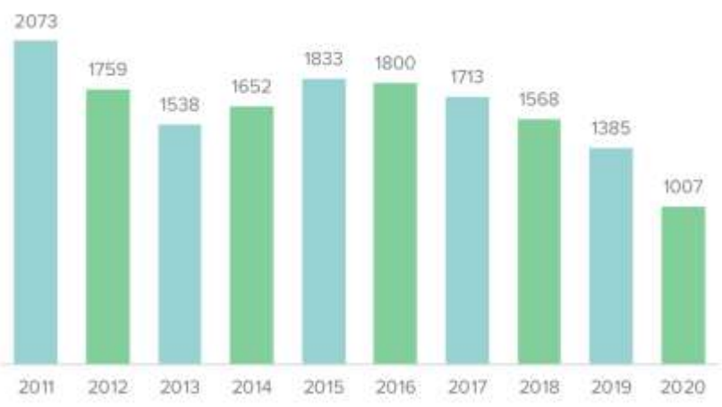
Número de homicidios de mujeres en Centroamérica y República Dominicana
