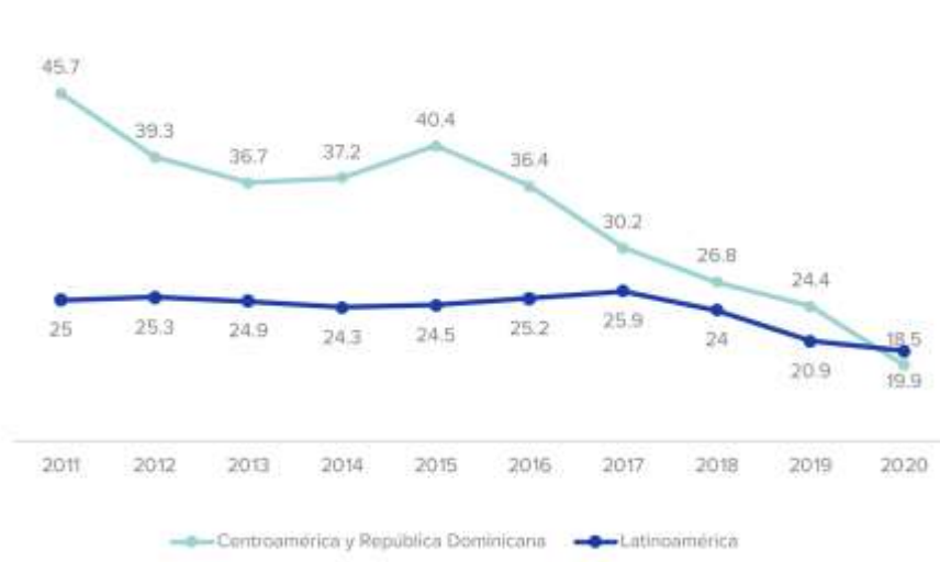
Tasas de homicidios de Centroamérica y República Dominicana vs Latinoamérica de 2010 a 2020 por cada 100 mil habitantes
