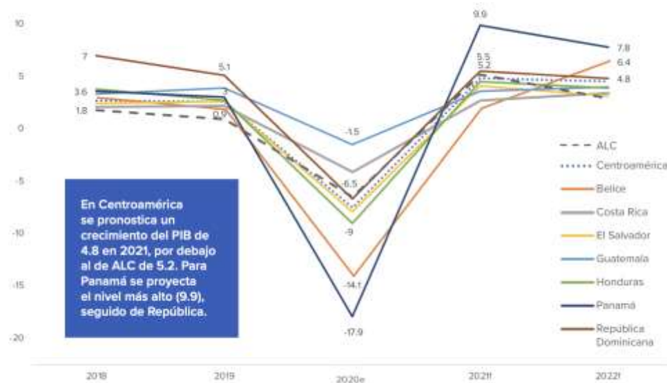
Pronósticos de crecimiento del PIB para la subregión. Años 2018-2022
