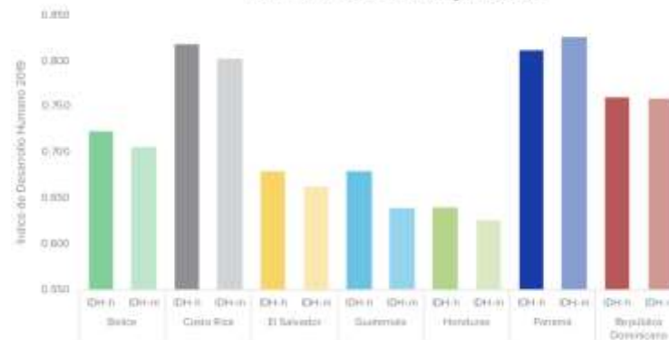
IDH hombres e IDH mujeres, 2019
