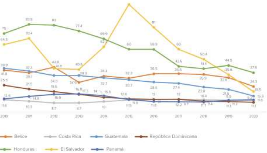
Tasas de homicidios por cada 100 mil habitantes por país
